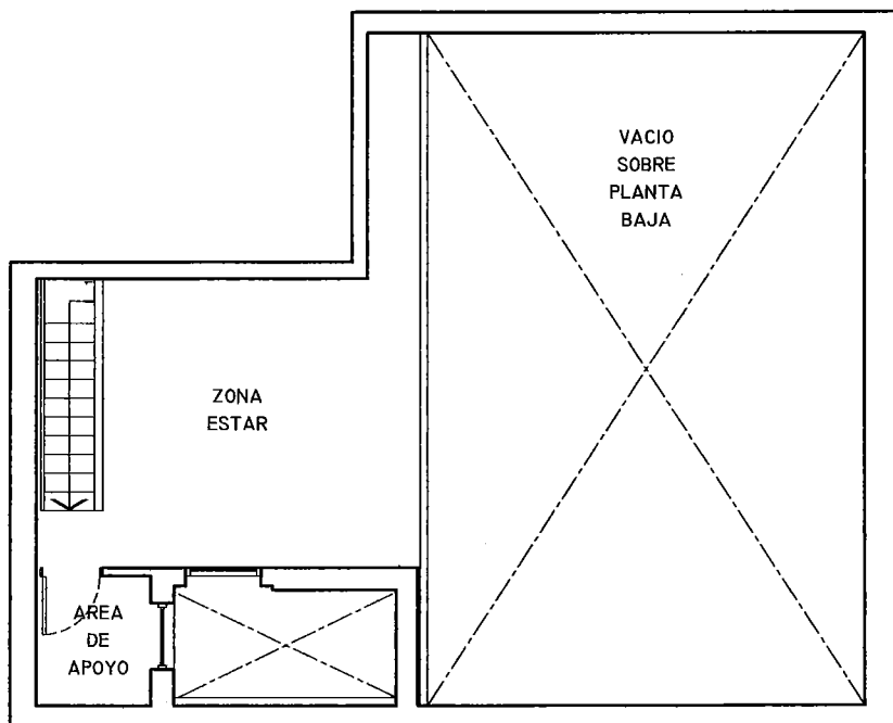
PLANTA ENTREPISO
